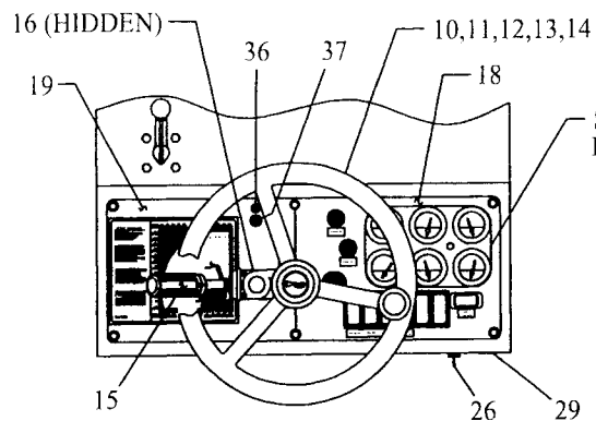
VIEW A-A
